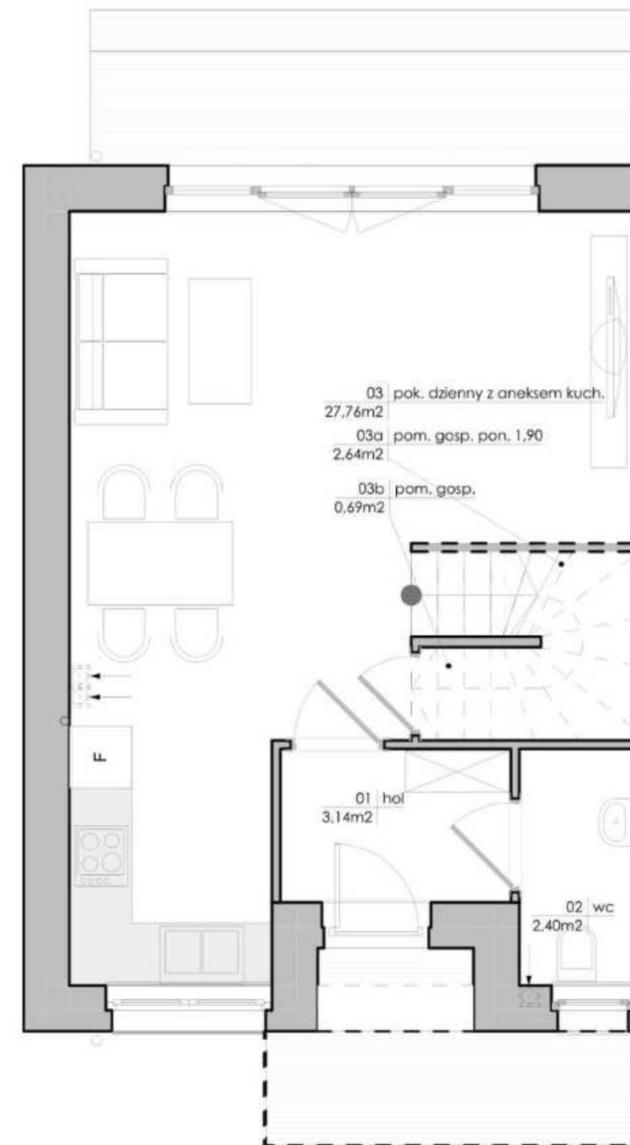
Mieszkanie - rzut parteru
