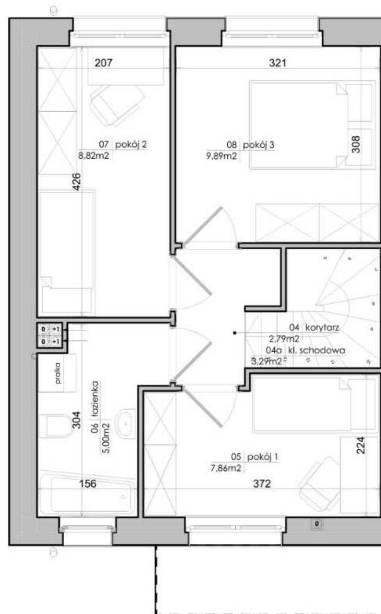
Mieszkanie - rzut piętra
