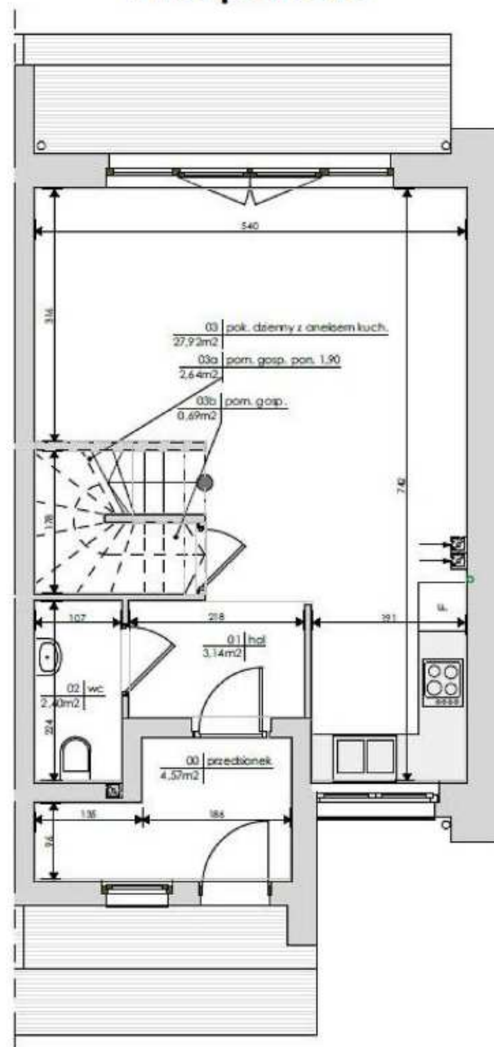
rzut parteru
